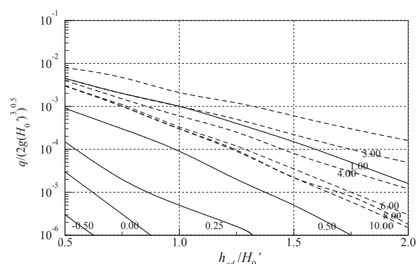
(b) 直立護岸：海底勾配 1/30，波形勾配 0.036
