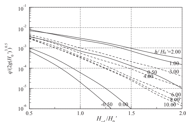
(d) 直立護岸：海底勾配 1/10，波形勾配 0.036
