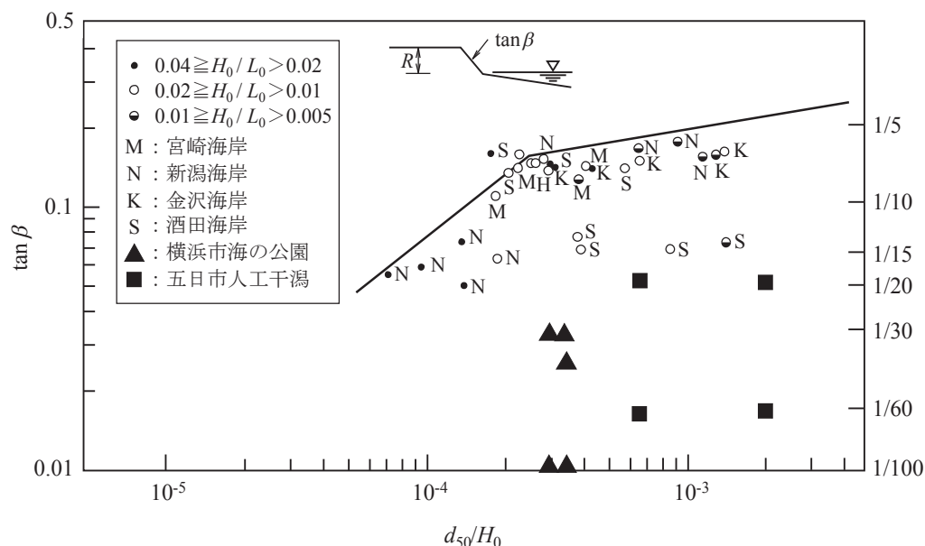
図-3.4.1 海底勾配と底質粒径との関係 4) ( \tan \beta は海底勾配、 d_{50} は中央粒径、 H_0 は沖波波高)
